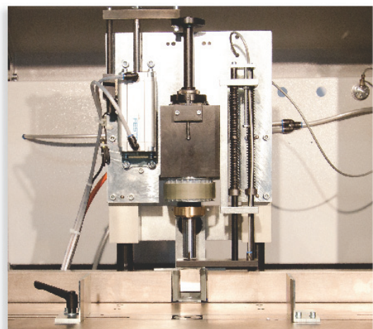
Bohrkopf für Daumenlochbohrung
